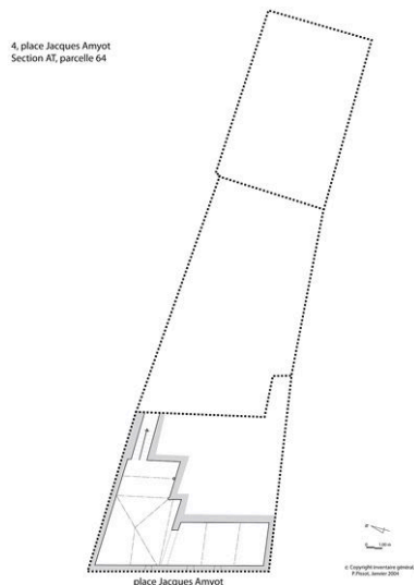
Plan de la cave médiévale. Dess. Pascal Pissot IVR11_20047700565NUD
