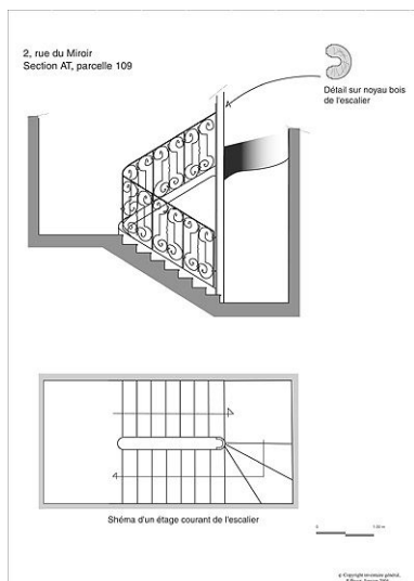
Plan et coupe de l'escalier en ferronnerie. Dess. Pascal Pissot IVR11_20047700619NUD
